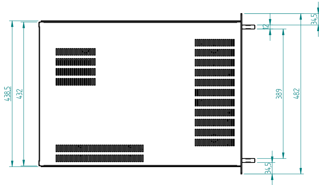
Appareil 5U
