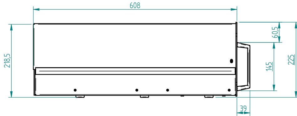
Appareil 5U
