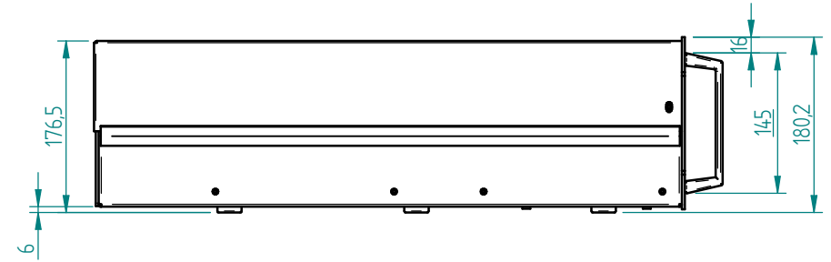
Appareil 4U
